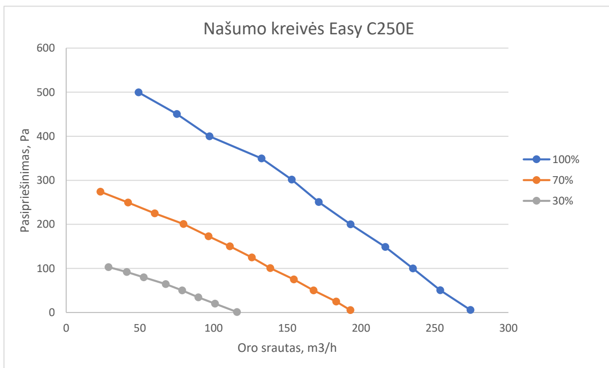
Grafikas 6 Vėdinimo galios priklausomybė nuo sumontuotos vėdinimo sistemos varžos
