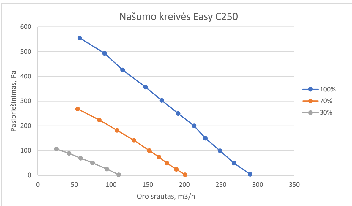
Grafikas 5 Vėdinimo galios priklausomybė nuo sumontuotos vėdinimo sistemos varžos
